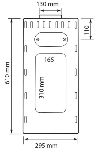
Sicht von oben top view
