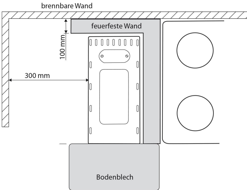
Abstand zu brennbaren Wänden - Sicht von oben Distance to combustible components - top view
